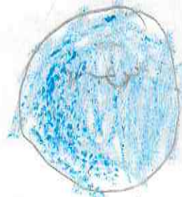
neptun
