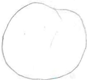
Uranus
