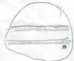
Jupiter
